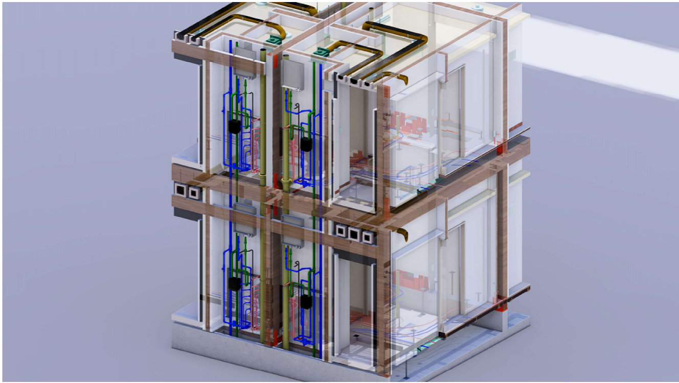
PS 部分パース (透過)
