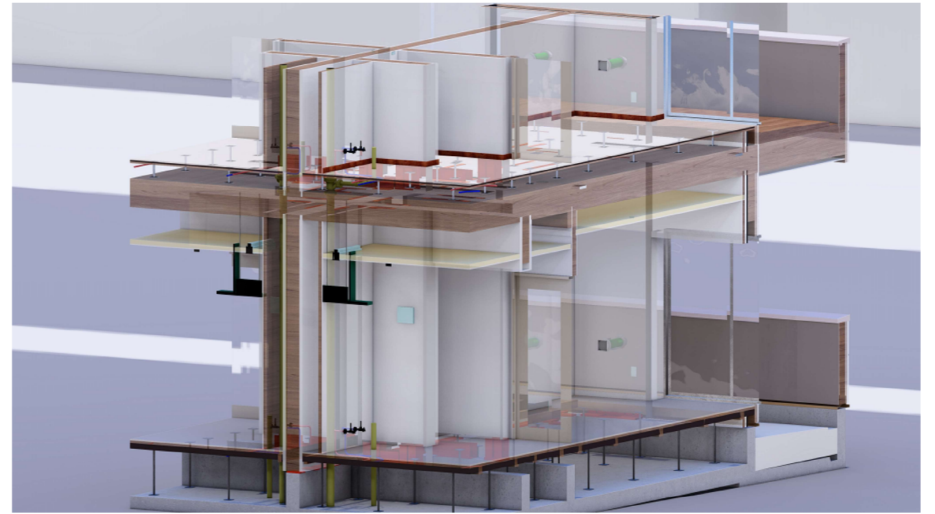
部分詳細（透過）
