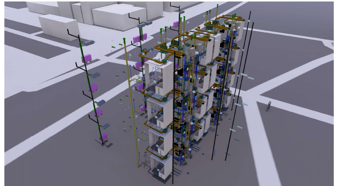
北東面
