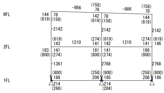
Y0 Y1 Y2 【 X6フレーム 】 S=1/250
