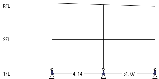
Y0 Y1 Y2 【 X2フレーム 】 S=1/250
