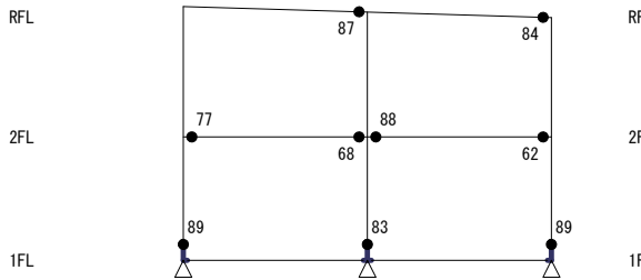
Y0 Y1 Y2 【 X0フレーム 】 S=1/250
