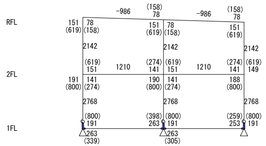
Y0 Y1 Y2 【 X1フレーム 】 S=1/250
