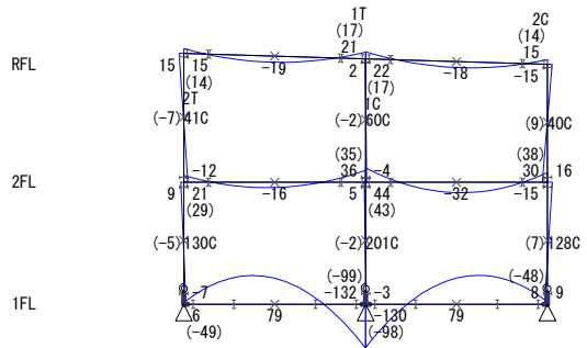
【 X1フレーム 】 S=1/250
