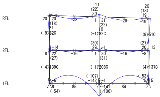
Y0 Y1 Y2 【 X4フレーム 】 S=1/250
