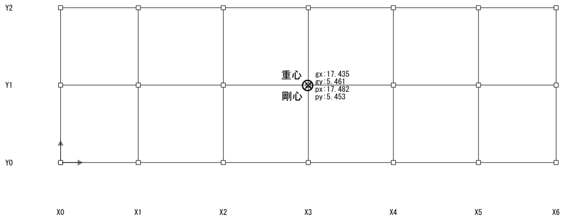
【 X正Y正 1F階 】
