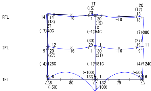
【 X2フレーム 】 S=1/250
