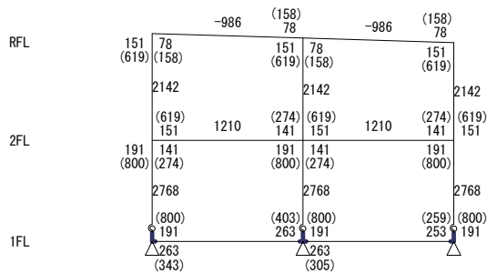
Y0 Y1 Y2 【 X2フレーム 】 S=1/250
