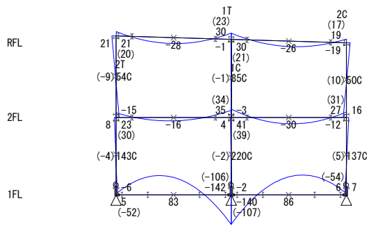
Y0 Y1 Y2 【 X5フレーム 】 S=1/250
