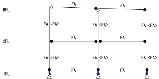
Y0 Y1 Y2 【 X1フレーム 】 S=1/250
