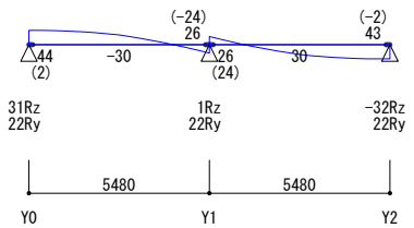
【 地震時Y方向負加力 】 S=1/250
