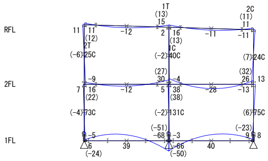
【 X0フレーム 】 S=1/250
