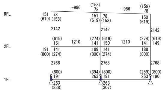
Y0 Y1 Y2 【 X5フレーム 】 S=1/250
