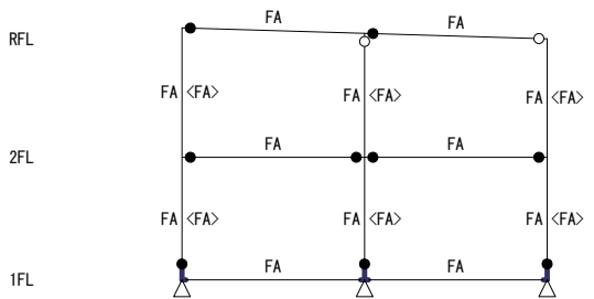
Y0 Y1 Y2 【 X2フレーム 】 S=1/250
