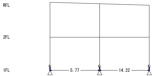
Y0 Y1 Y2 【 X0フレーム 】 S=1/250
