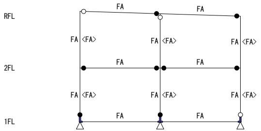
Y0 Y1 Y2 【 X0フレーム 】 S=1/250
