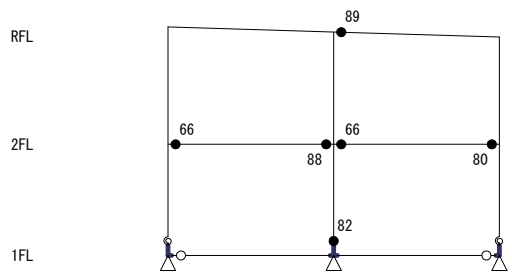
Y0 Y1 Y2 【 X6フレーム 】 S=1/250
