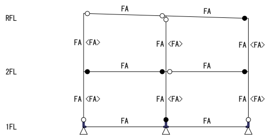
Y0 Y1 Y2 【 X6フレーム 】 S=1/250
