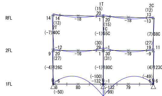
【 X3フレーム 】 S=1/250
