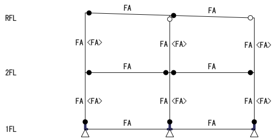
Y0 Y1 Y2 【 X3フレーム 】 S=1/250
