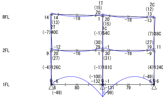
【 X4フレーム 】 S=1/250
