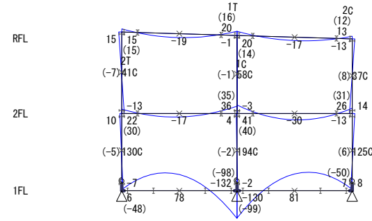
【 X5フレーム 】 S=1/250
