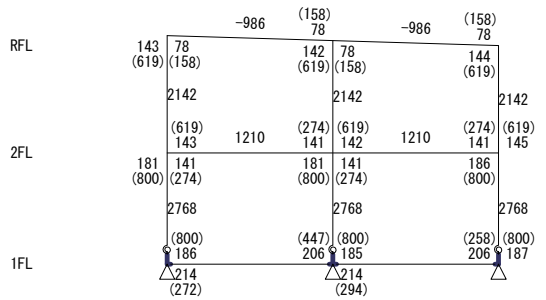
Y0 Y1 Y2 【 X0フレーム 】 S=1/250
