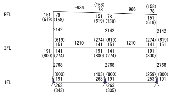
Y0 Y1 Y2 【 X3フレーム 】 S=1/250
