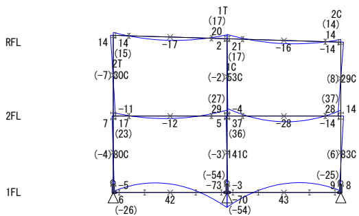
Y0 Y1 Y2 【 X6フレーム 】 S=1/250
