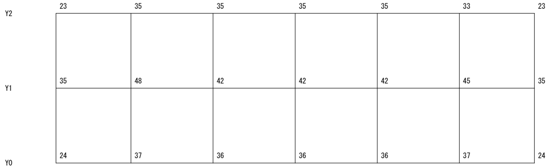
X0 X1 X2 X3 X4 X5 X6 【 RFL層 】 S=1/270
