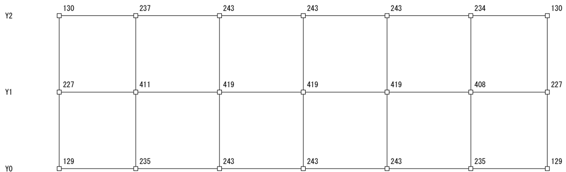
X0 X1 X2 X3 X4 X5 X6 【 2FL層 】 S=1/270
