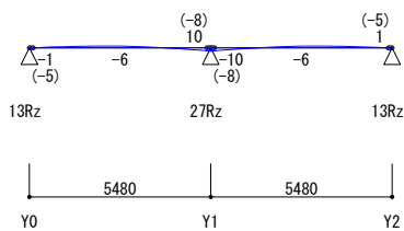
【 短期積雪時 】 S=1/250
