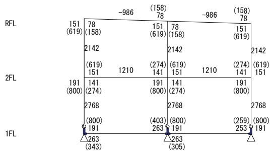
Y0 Y1 Y2 【 X4フレーム 】 S=1/250
