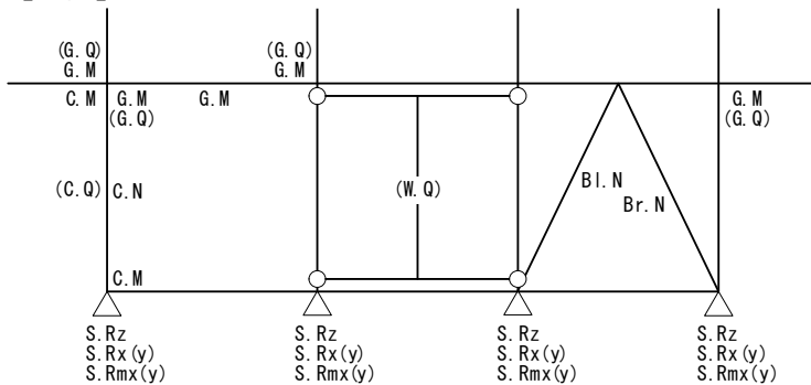
中間荷重がかからない場合
