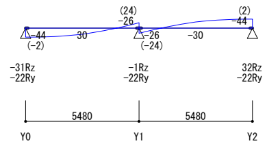
【 地震時Y方向正加力 】 S=1/250
