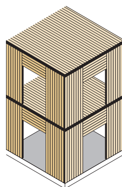
CLTパネル工法
