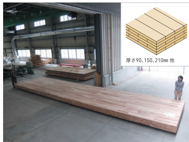
現在、国内で製造可能な最大のCLTパネル(幅3m×長さ12m、銘建工業)
