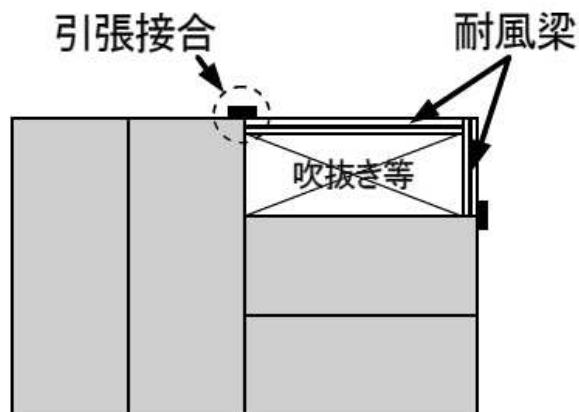
図 2：耐風梁および引張接合部の配置例
