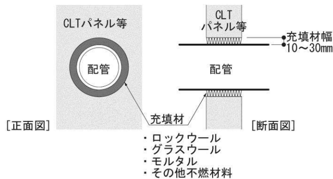
図 1 配管・配線の場合
