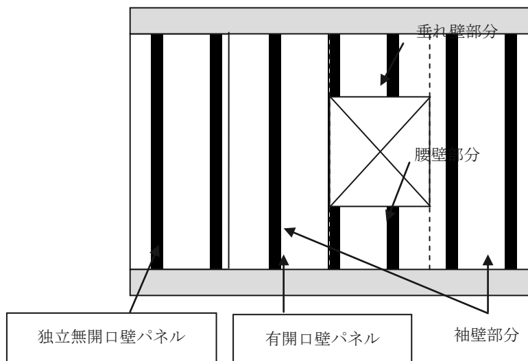
図2-7：各パネルの外層ラミナ方向
