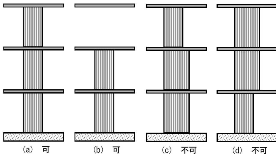
図 1－2：上下階の耐力壁配置
