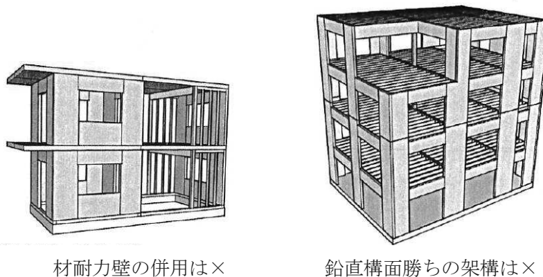
図1：「ルート1パネル工法」とならない建築物の例
