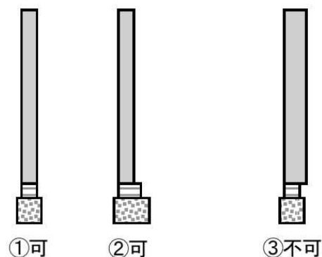
図1：土台の幅と壁パネル厚さの関係
