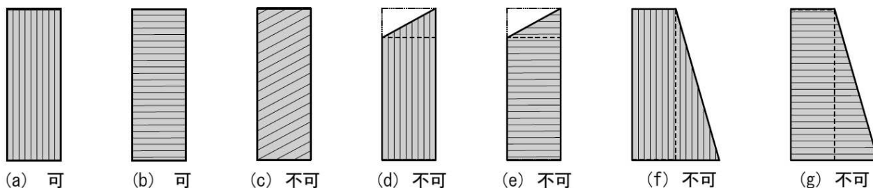
図 1－8：壁パネルの形状と外層ラミナ方向の関係
