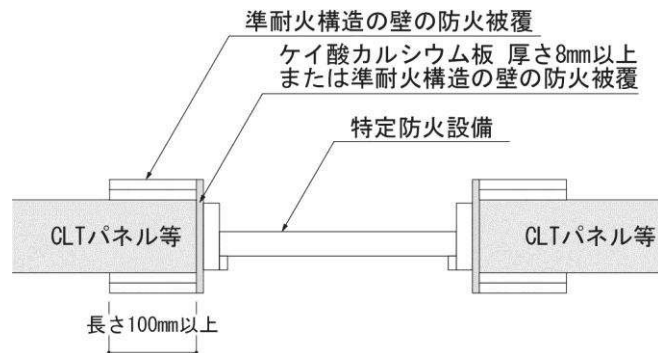
図 1：サッシ・扉等開口部の防火措置
