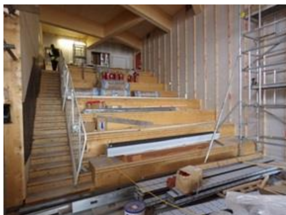
写真 9-3 屋内エントランス階段（CLT）
