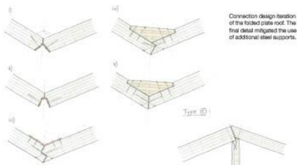
図 3-6 屋根部分の接合のイラスト*3
