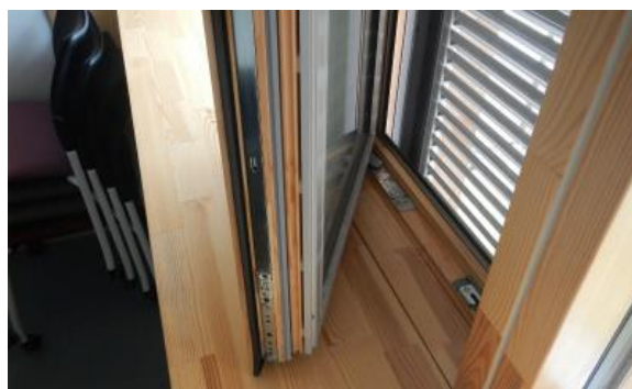
写真 7-4 トリプルガラスのサッシ
