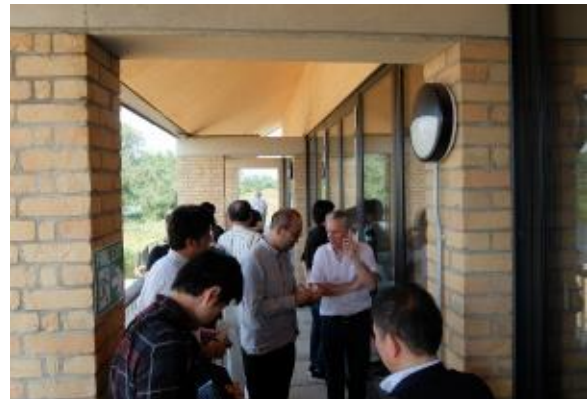
写真 11-4 北側ベランダ（ベランダの天井は CLT が現し、RC の梁との接合金物も見えている）
