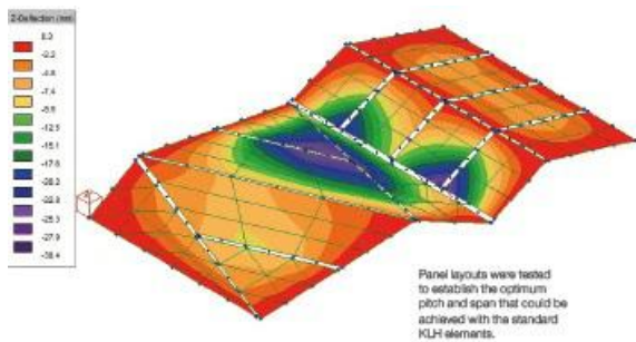
図 3-2 屋根パネルの構造解析図*3
