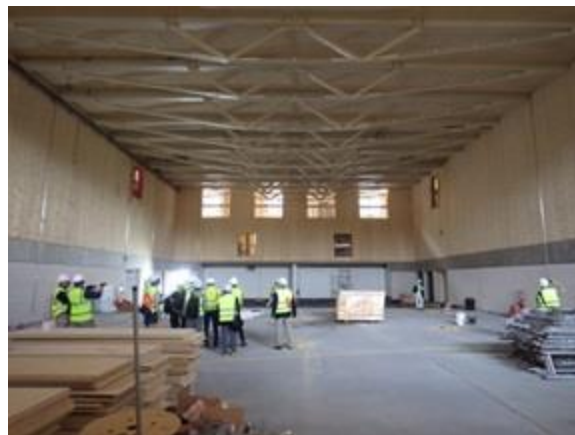
写真 9-4 半地下の屋内運動場
