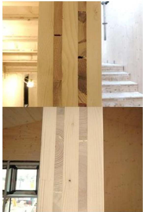
写真 3-13, 14 CLT 壁の木口断面 (下段では幅はぎすき間に現場でパテ埋め)
