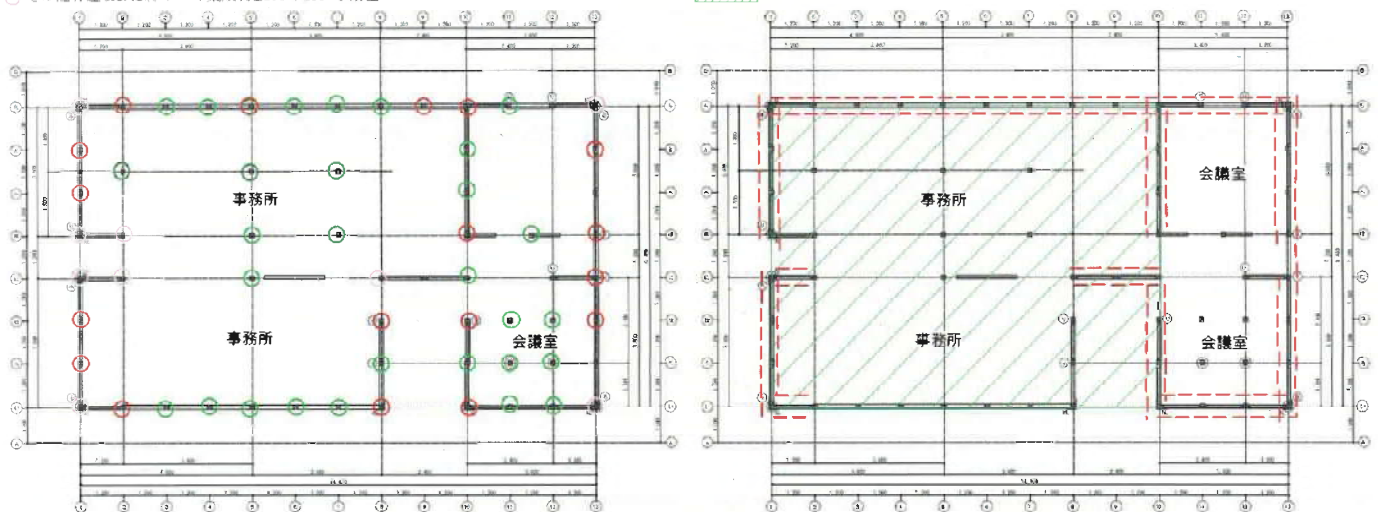
図 軸組工法等の平面図の例
