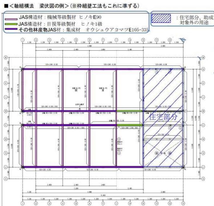
図1-3 軸組工法等の梁伏図の例
