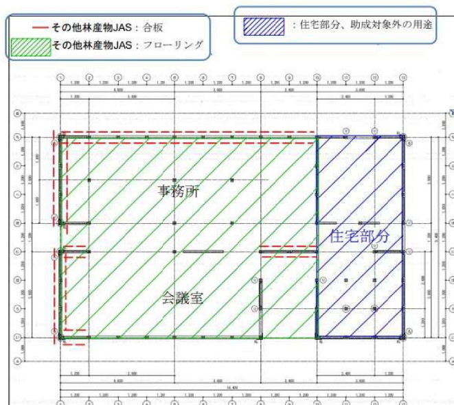
■&lt;軸組構法 平面図の例&gt;(※軸組壁工法もこれに準ずる)
