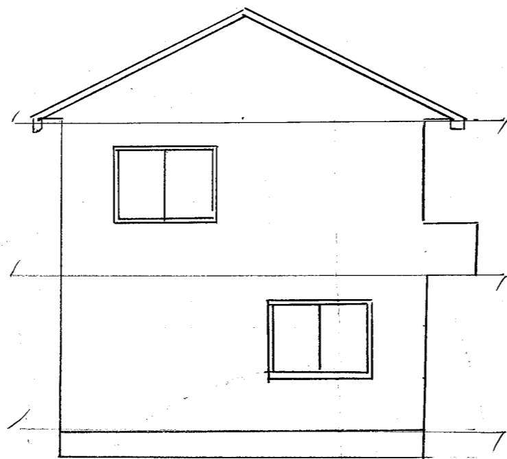
西面
